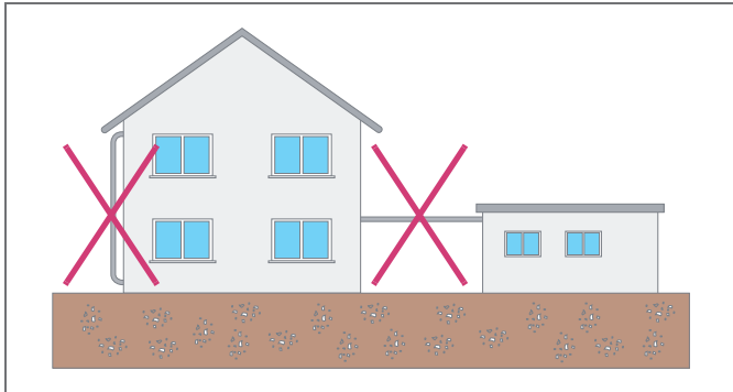
Rys. 18-5 Montaż rur poza budynkiem jest dopuszczalny tylko pod warunkiem zastosowania odpowiednich środków ochronnych
