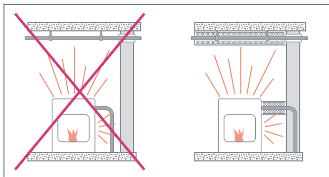
Rys. 18-3 Ochrona przed nadmiernym ogrzewaniem rur
