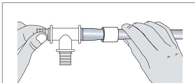
Rys. 11-7 Wsunąć złączkę w rozszerzony koniec rury
