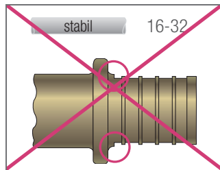
Rys. 7-10 Złączka mosiężna, pierścień oporowy częściowo uformowany, zakres średnic 16–32
