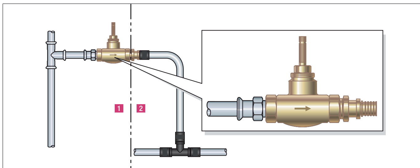
Rys. 7-27 Przykład montażowy połączenia systemów instalacyjnych z innych materiałów poprzez zawór podtynkowy
