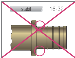
Rys. 7-9 Złączka mosiężna, brak pierścienia oporowego, zakres średnic 16–32
