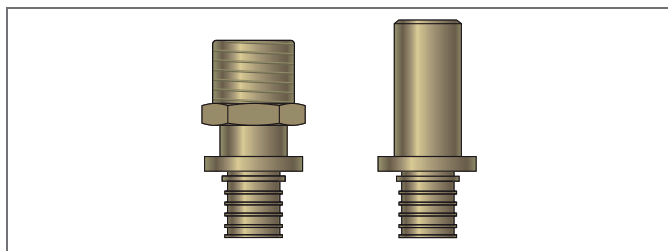
Rys. 7-20 Złączki RAUTITAN MX do przejścia na inne materiały
