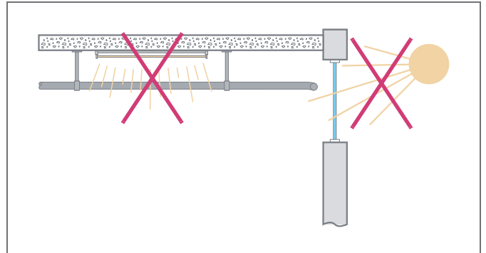
Rys. 18-7 Montaż rur w obszarze działania promieni UV bez odpowiedniej ochrony jest niedopuszczalny – przykład instalacji wewnątrz budynku
