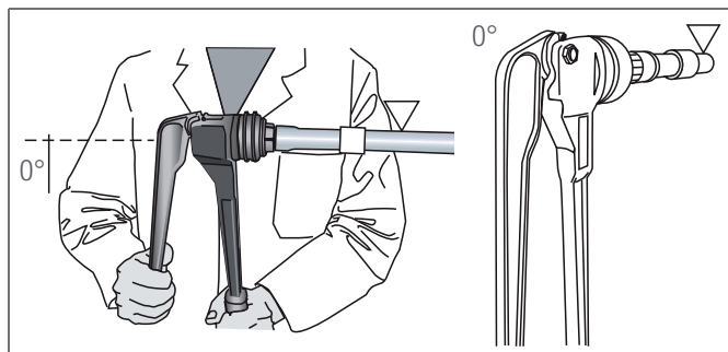
Rys. 11-5 Kielichowanie rury
