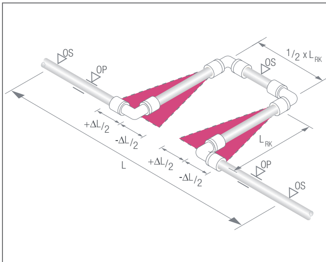
Rys. 17-2 Łuk wydłużający U
