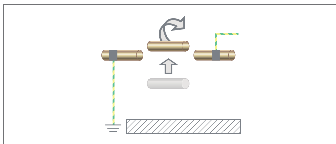
Rys. 18-12 Wyrównanie potencjałów przy wymianie rur
