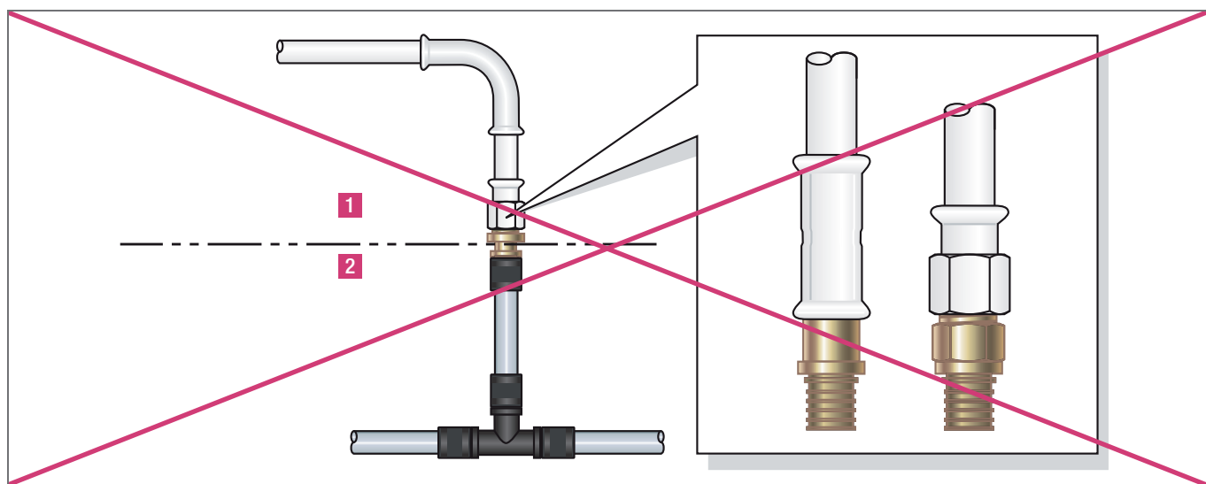
Rys. 7-29 Przykład montażowy niepoprawnego połączenia systemu RAUTITAN z systemem ze stali nierdzewnej o średnicy 32 lub gwintem do R1/Rp1.
