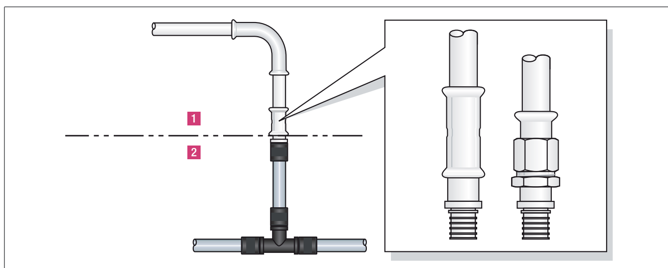
Rys. 7-28 Przykład montażowy bezpośredniego połączenia systemu RAUTITAN z systemem ze stali nierdzewnej do średnicy 32 lub gwintem do R1/Rp1 ze stali nierdzewnej.
