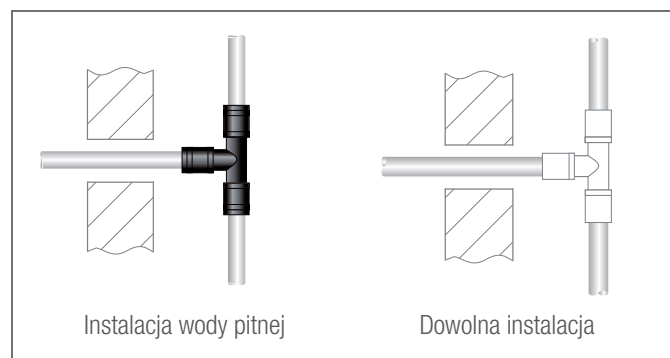
Rys. 1-1 Przykład instalacji wody pitnej (po lewej) oraz przykład obejmujący różne systemy (po prawej)
